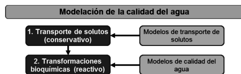
Figura 3. Esquematización de la relación entre la modelación del transporte de solutos (conservativo) y de las transformaciones bio-químicas (reactivo).
